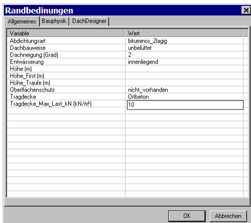
Bild 1.4: Randbedingungen
