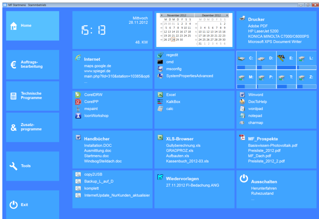
Bild: Muster-Home-Bildschirm
