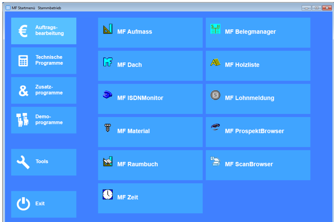
Bild: Startbildschirm
