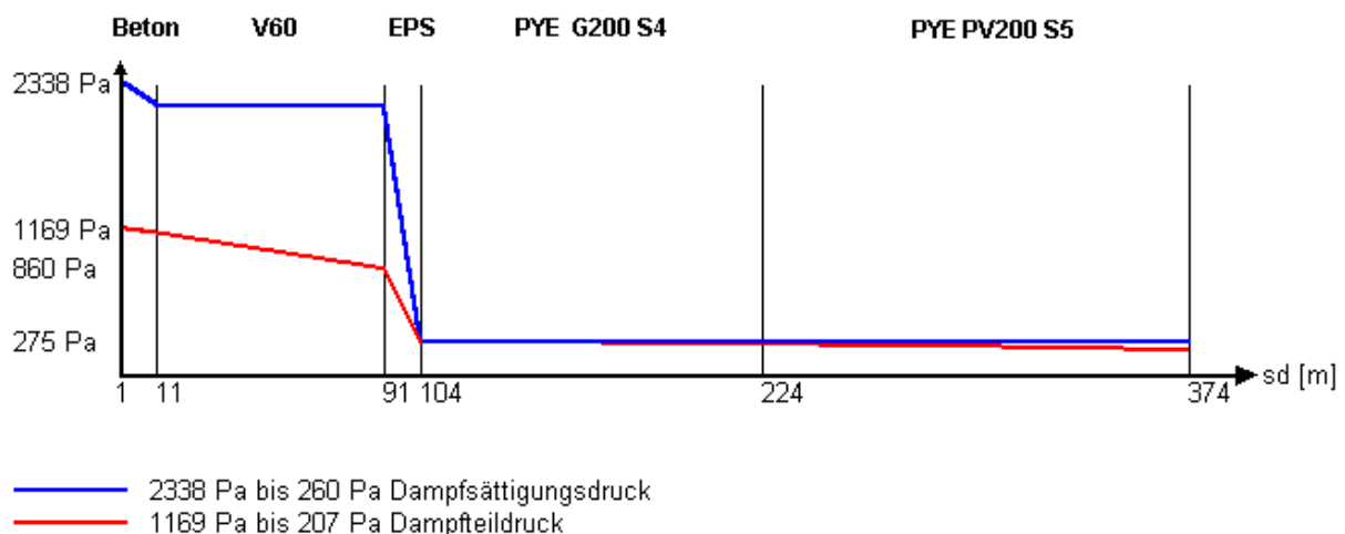
Abbildung 4: Glaserdiagramm Warmdach
