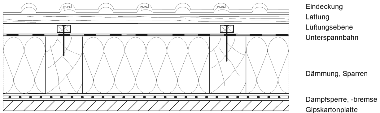
Abbildung 3: Sparrendach
